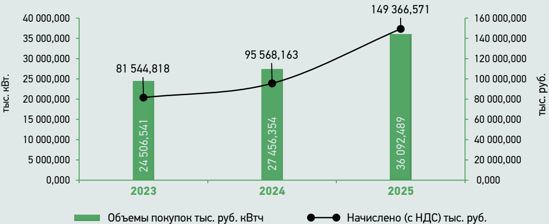
Изменение объемов и стоимости покупной электроэнергии (мощности) на ОРЭМ за последние 3 года:
