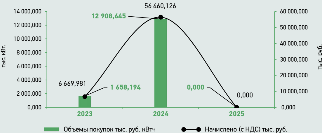
Изменение объемов и стоимости покупной электроэнергии (мощности) на РРЭ за последние 3 года:
